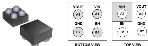
0.77 mm x 0.77 mm x 0.35 mm Thin WLCSP
